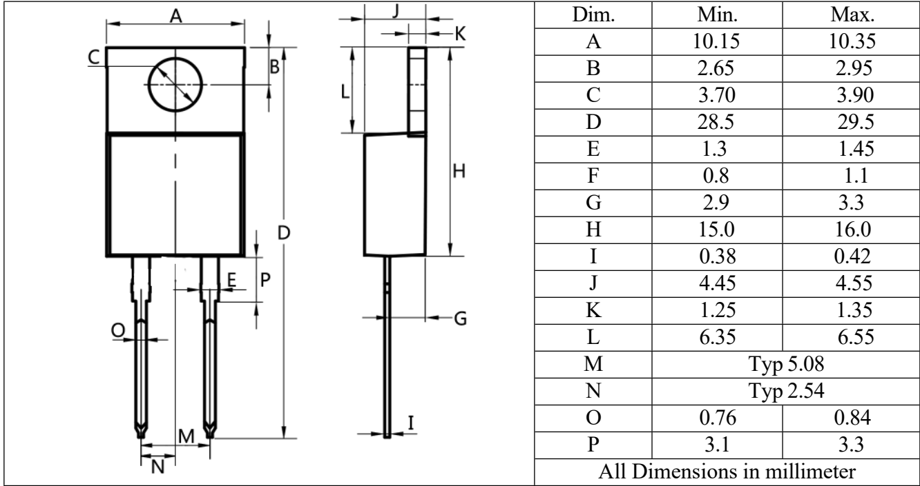
TO-220AC 封装尺寸 Package size
