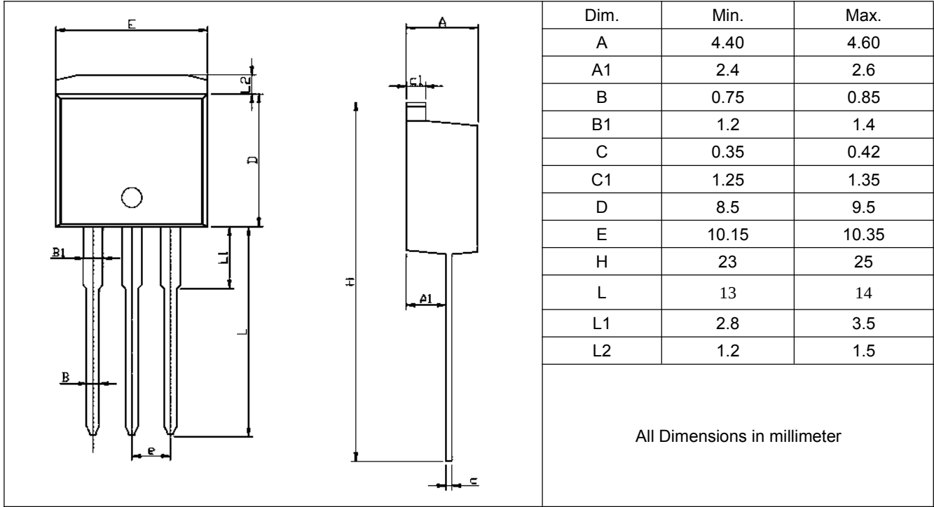
TO-262 封装尺寸 Package size
