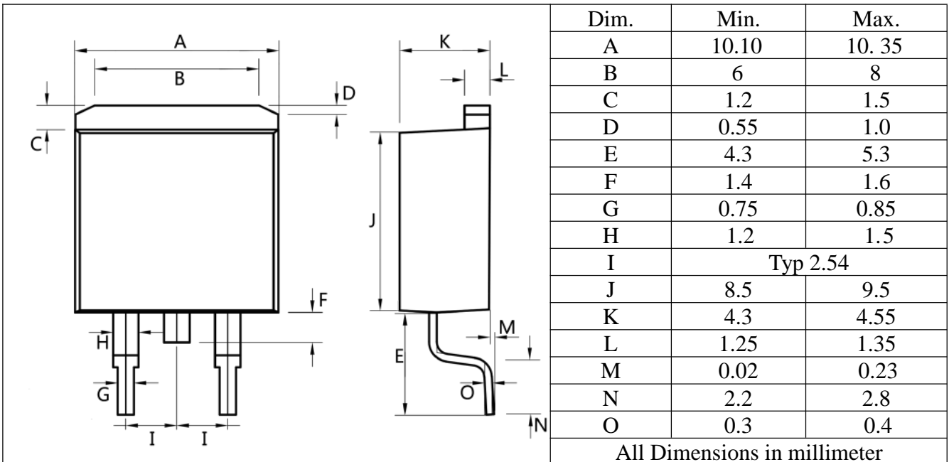
TO-263 封装尺寸 Package size
